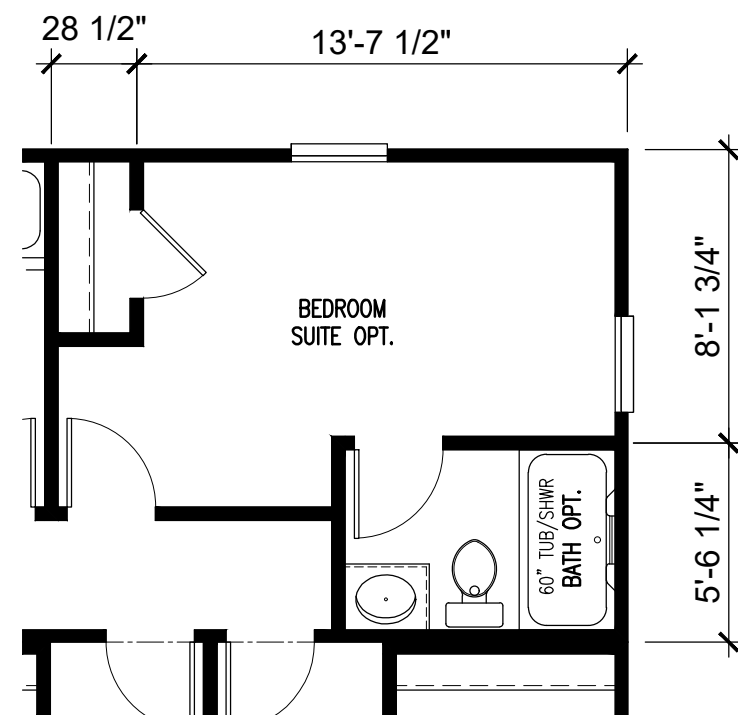
BEDROOM 4 SUITE OPTION
